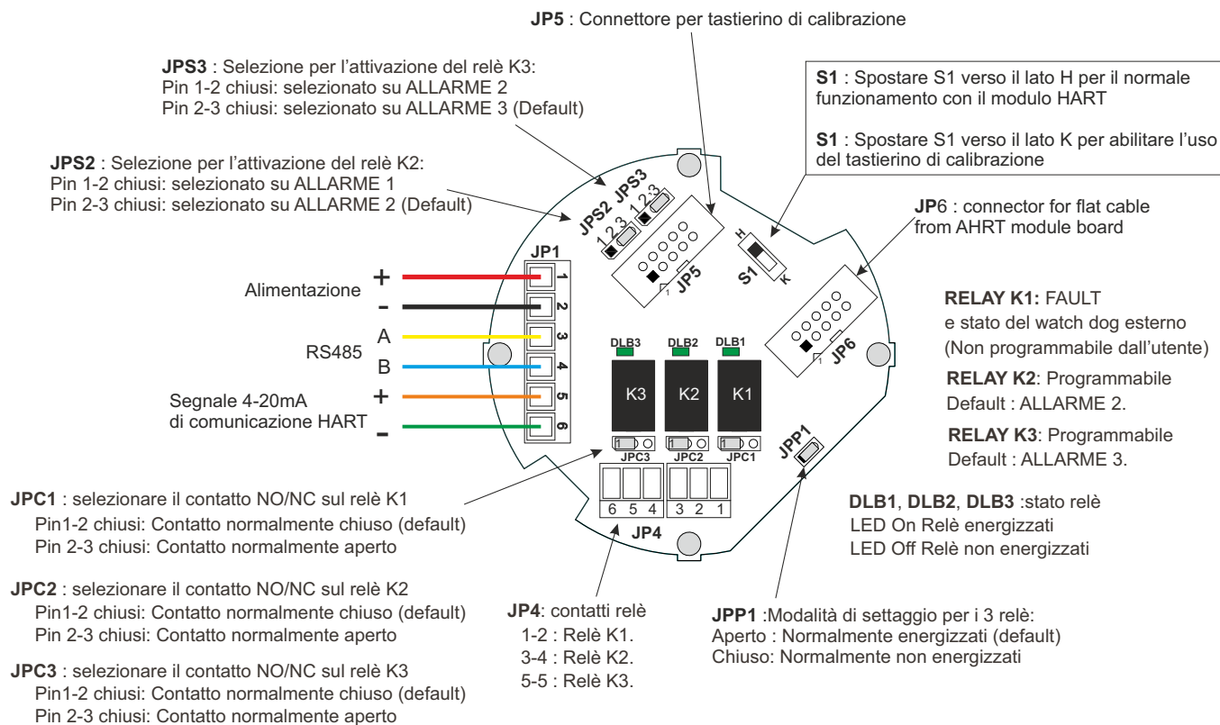
Figura 1) Schema topografico della scheda base senza modulo HART
