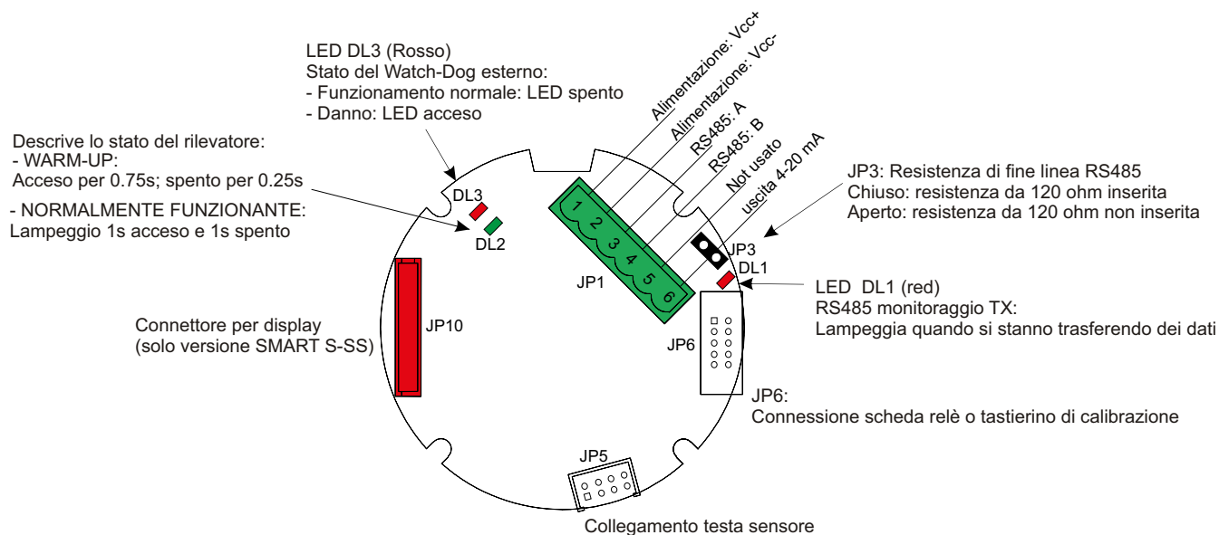
Figura 2) Schema topografico della scheda base equipaggiata con modulo HART
